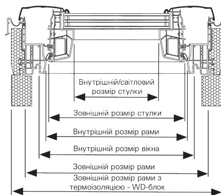
поперечний переріз для ПВХ
